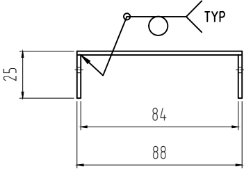
KT-9 VL: Thép tấm A240 304-2mm SL: 2-Scale 3:1
