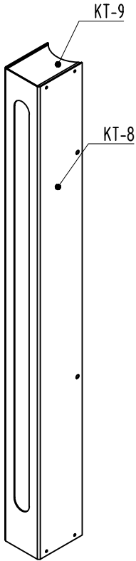
KT-8.2 VL: Thép tấm A240 304-2mm SL: 1
