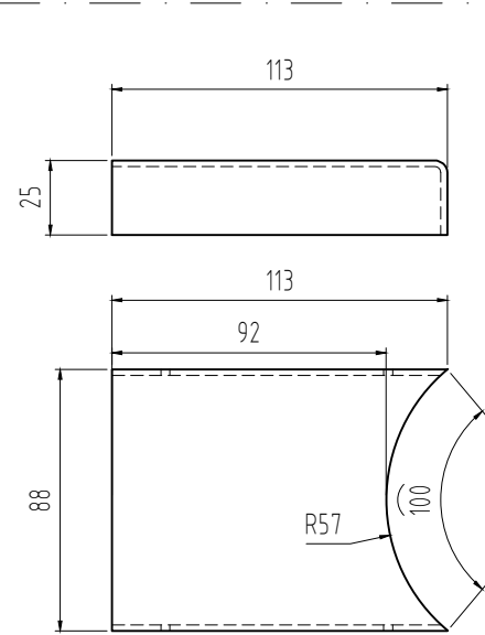
KT-9 VL: Thép tấm A240 304-2mm SL: 2-Scale 3:1
