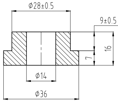
P18.4 SUS304-16mm Q'ty:01
