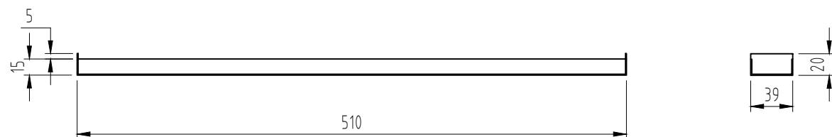
P21.2 A240 304-2mm Q'ty:128
