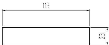
KT-9.2 VL: Thép tấm A240 304-2mm SL: 4-Scale 3:1
