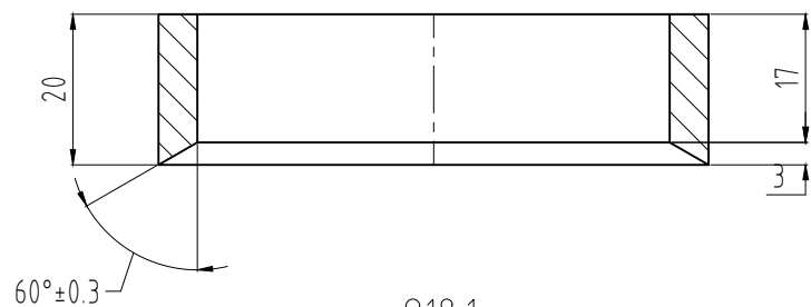
O18.1 A312 TP304, \phi 76 \times 5.16 \text{ mm} SL:01
