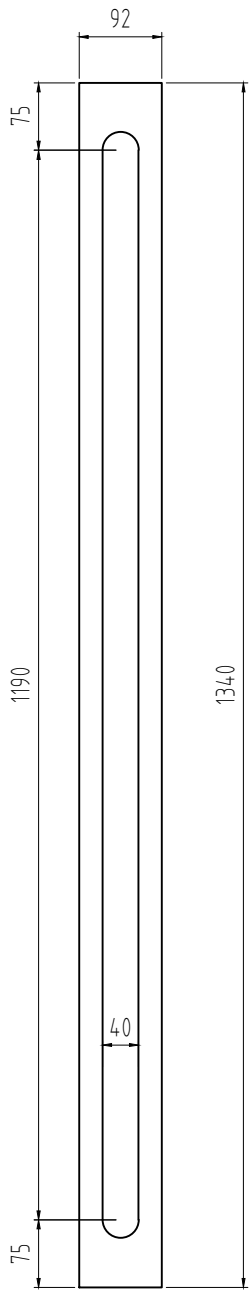
KT-8.2 VL: Thép tấm A240 304-2mm SL: 1
