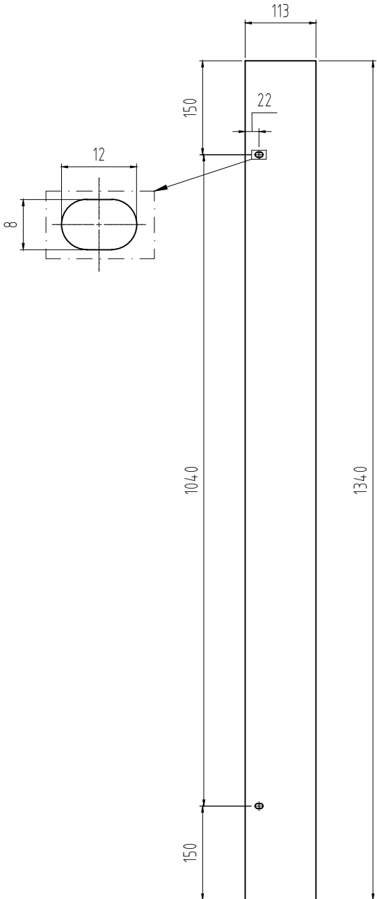
KT-8.1 VL: Thép tấm A240 304-2mm SL: 2
