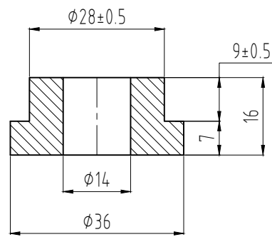
P18.4 SUS304-16mm Q'ty:01
