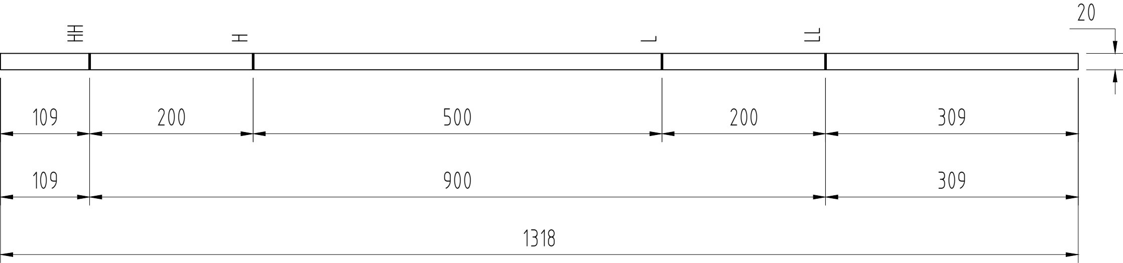
KT-18(Thước chia mức nước) SL: 2
